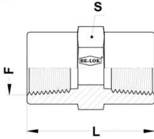
Fig.-A SAE 140138
